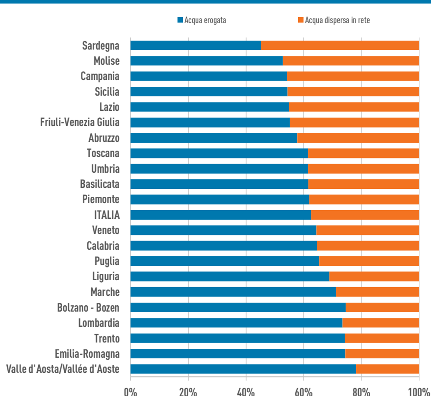
FIGURA 7. Acqua erogata e dispersa nelle reti comunali di distribuzione dell'acqua potabile per regione. Anno 2012. Valori percentuali sul totale di acqua immessa
