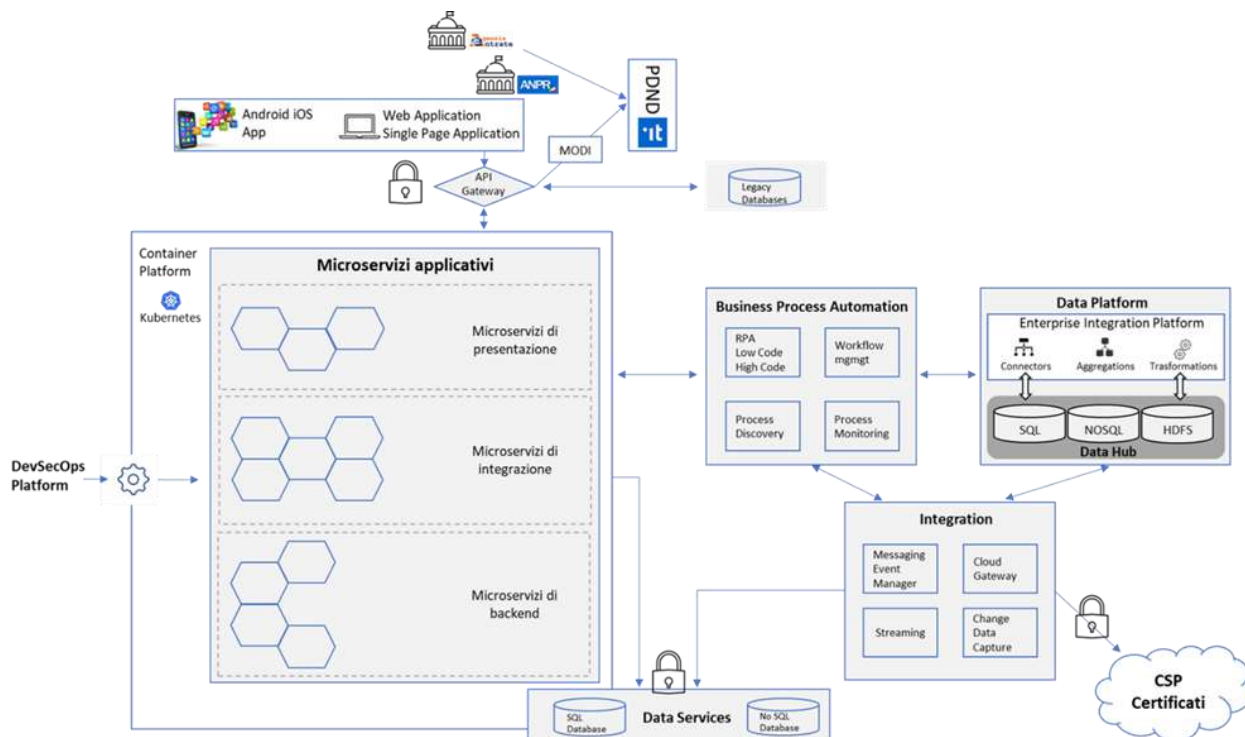
Figura 8 - Esempio di modello fisico di riferimento
