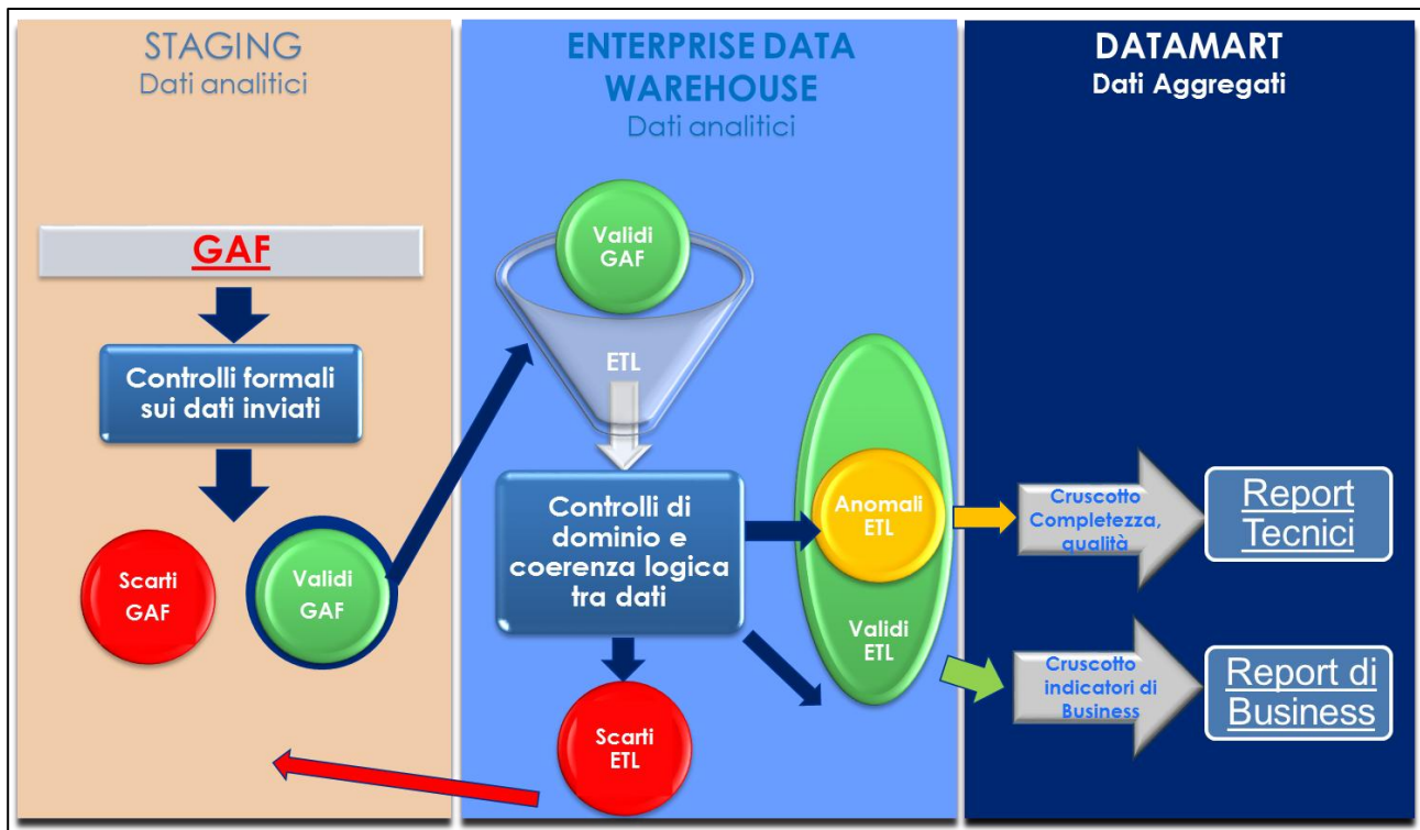
Figura 2.2.1 - Il processo di acquisizione dei dati
