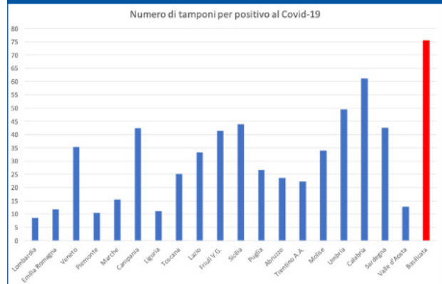
Figura 8. Numero di tamponi rinofaringei effettuati in Basilicata e sottoposti a PCR per l'estrazione dell'RNA del virus SARS-CoV-2 alla data del 31 maggio 2020 rapportato al numero di casi positivi (7)
