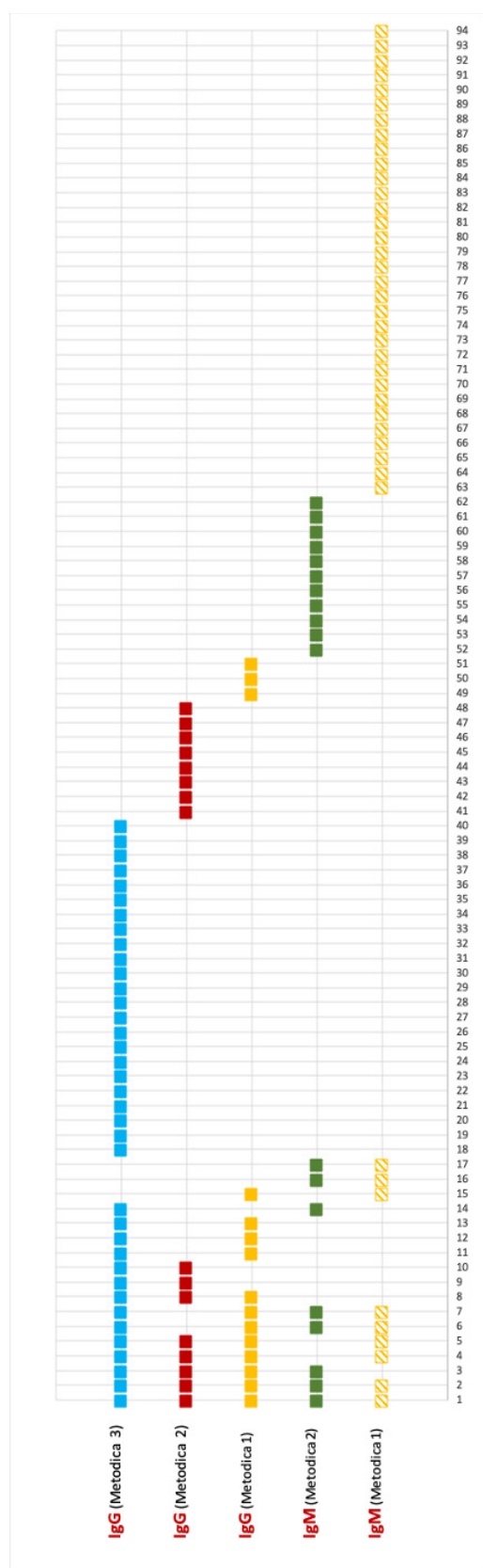
Figura 6. Risultati delle metodiche sierologiche sul campione di popolazione coinvolto nello screening
